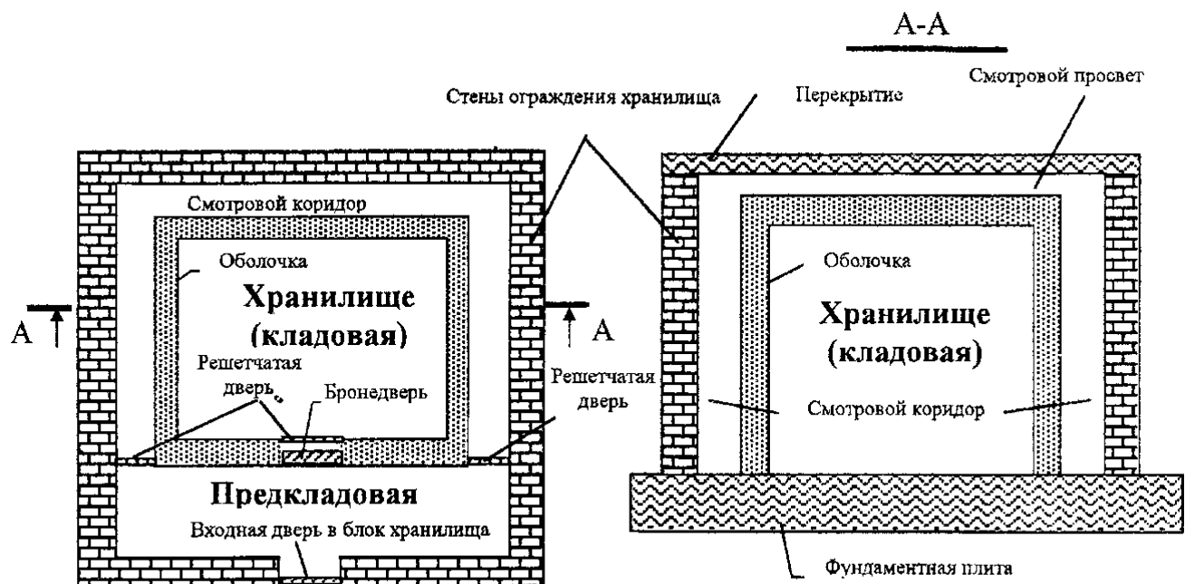
Рисунок П8.1- Схематическое устройство хранилища ценностей
